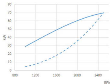
Puissance (ISO 3046/1)
