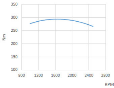
Couple au vilebrequin
