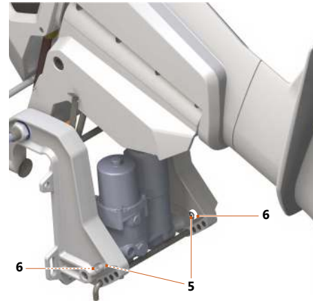
Abb. 29: Opferanoden Spiegelhalterung
