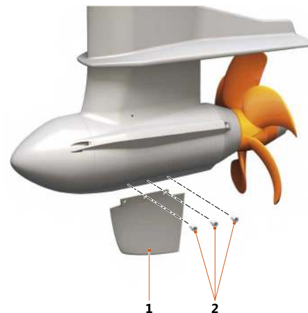
Abb. 7: Finnenbefestigung
