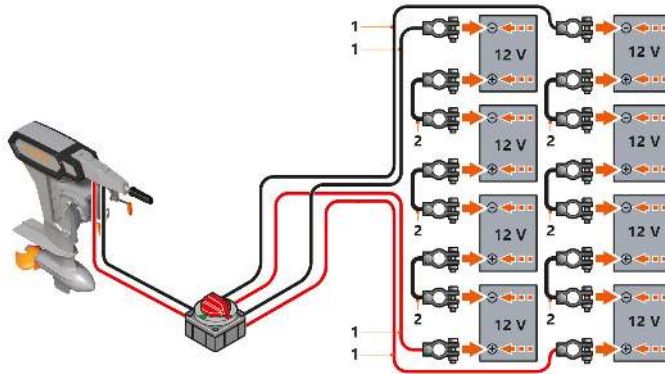
Abb. 12: Schaltplan Bleibatterien
