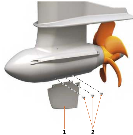
Abb. 27: Finnenbefestigung
