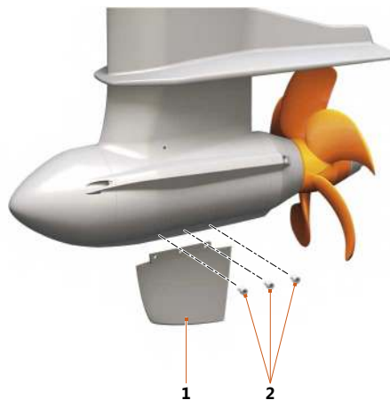
Fig. 58: Fin attachment
