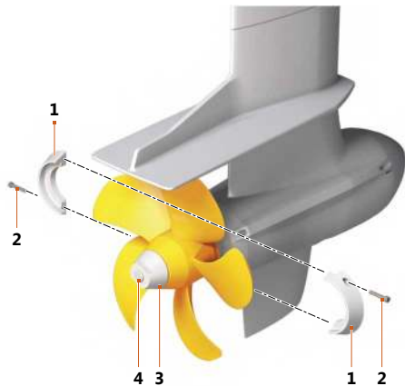
Fig. 59: Anodes
