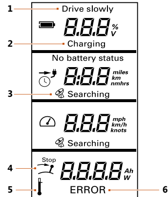
Abb. 15: Multifunktionsanzeige Setup-Menü
