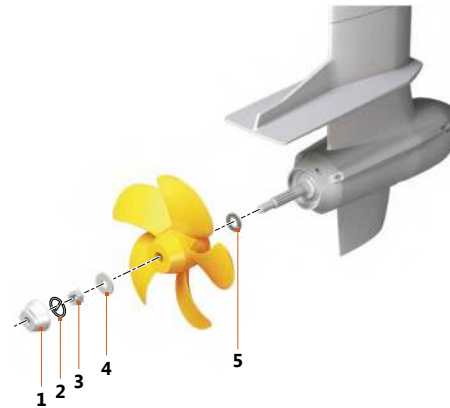
Abb. 26: Propellerbefestigung
